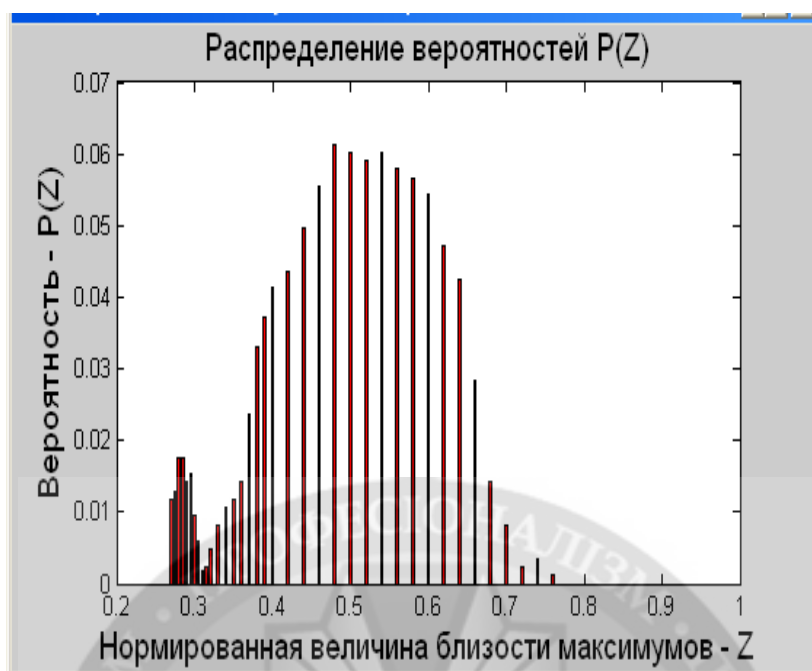
Рис. 1. Плотность вероятности меры близости Z для записи двух ЦФ на одной АЦЗЗ
